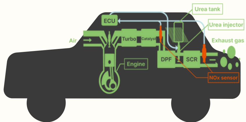
車輛-引擎排氣 示意圖
